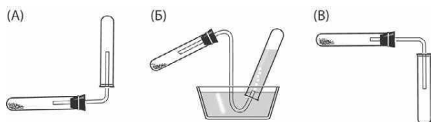
Рис. 7. Приборы для собирания газов
